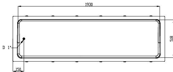
Boven aanzicht
